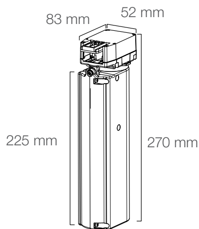
Wymiary napędu przesuwu zasłon
